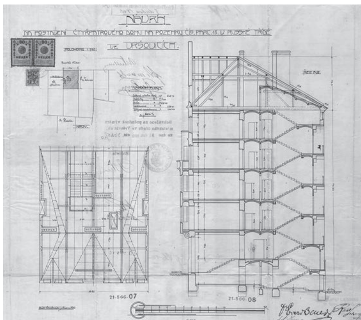
Příčný řez domem manželů Benešových ve Vršovicích.
